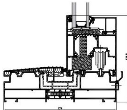
MB-77HS HI
