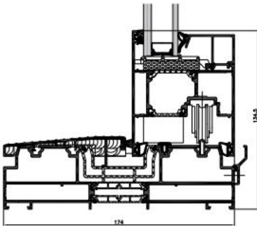
MB-77HS ST
